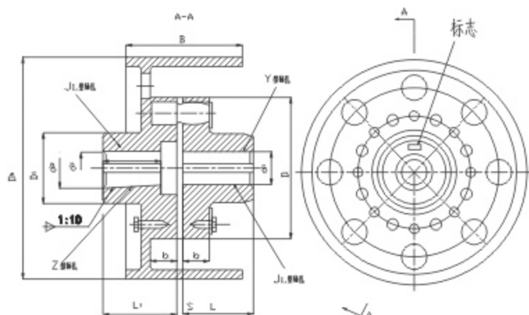
LXZ(HLL)型带制动轮弹性柱销联轴器主要参数与尺寸
