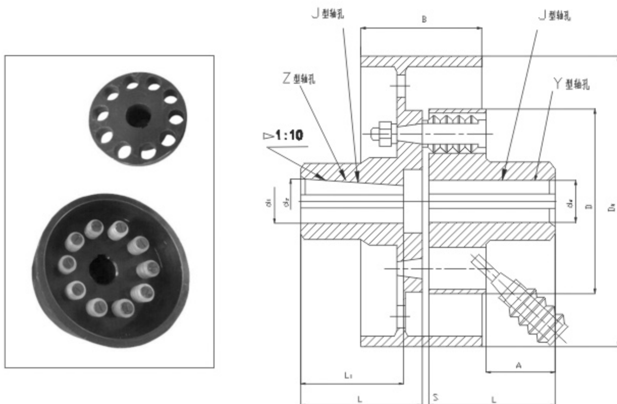
LTZ型联轴器主要参数与尺寸 (GB/T 4323-2002)
