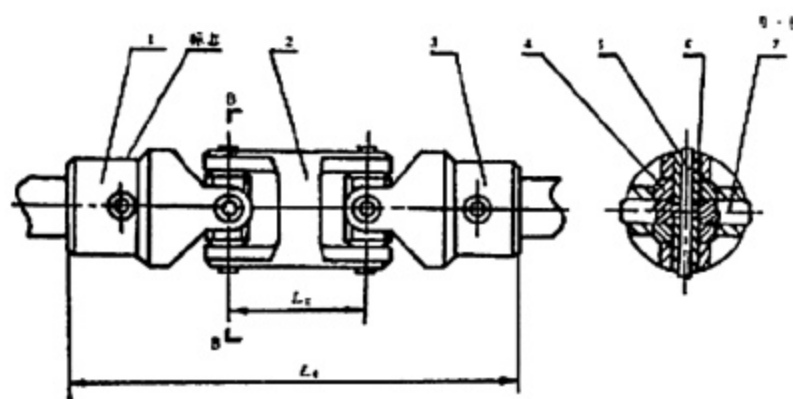
图2 WS型双十字轴万向联轴器
